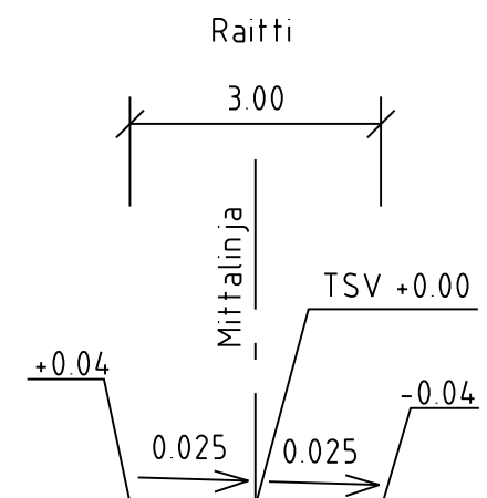
TYYPPIPOIKKILEIKKAUS A-A 1:200
