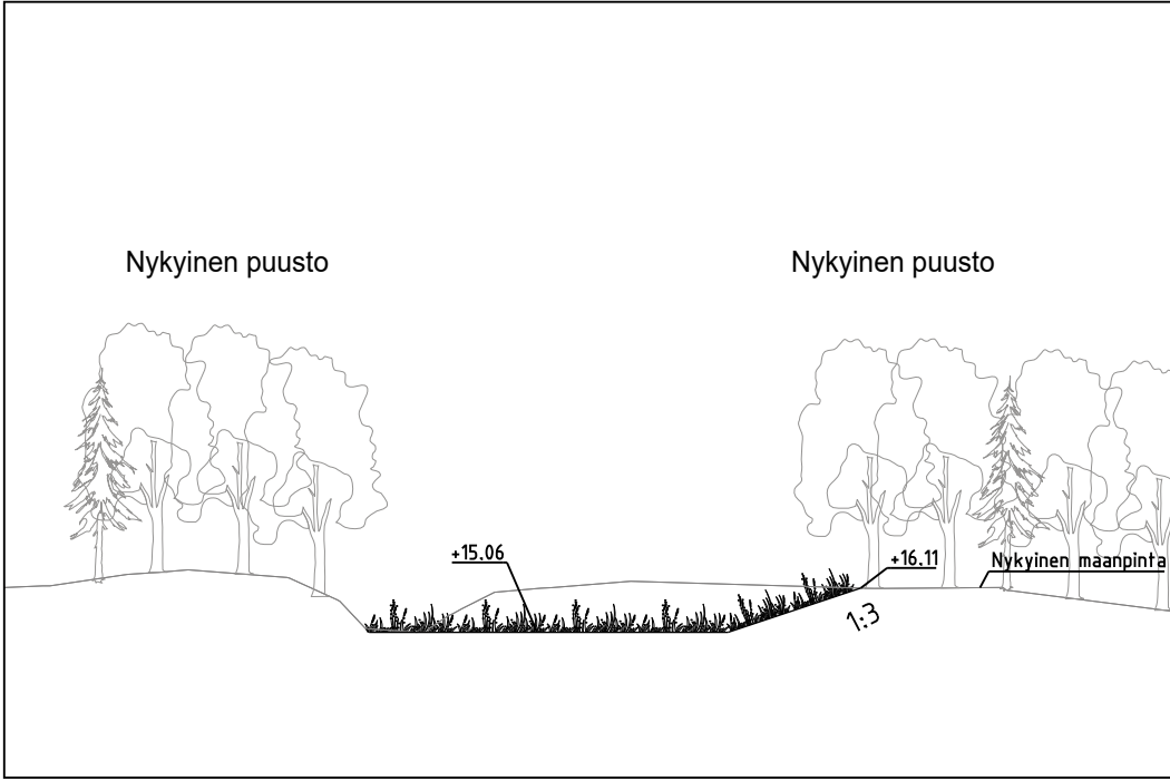
TYYPPIPOIKKILEIKKAUS B-B, 1:200
