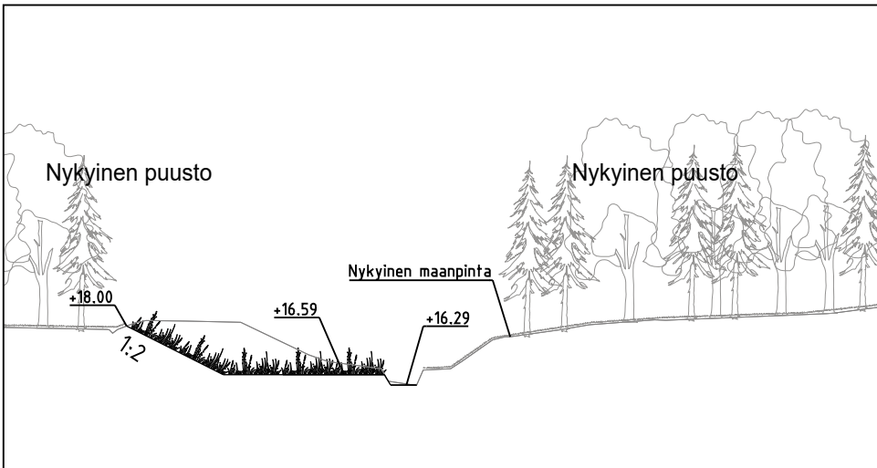
TYYPPIPOIKKILEIKKAUS A-A, 1:200
