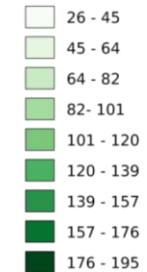
MS-NFI-2019, mean volume, m³/ha
