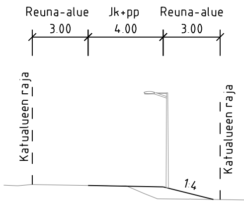
TYYPPIPOIKKILEIKKAUS E-E 1:200
