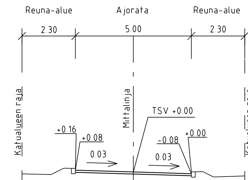
TYYPPIPOIKKILEIKKAUS A-A 1:200
