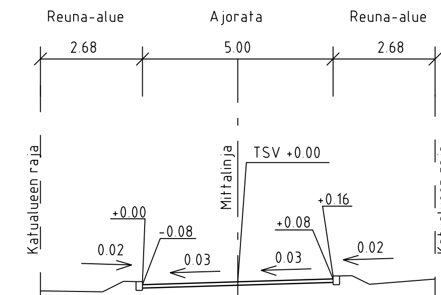
TYYPPIPOIKKILEIKKAUS B-B 1:200
