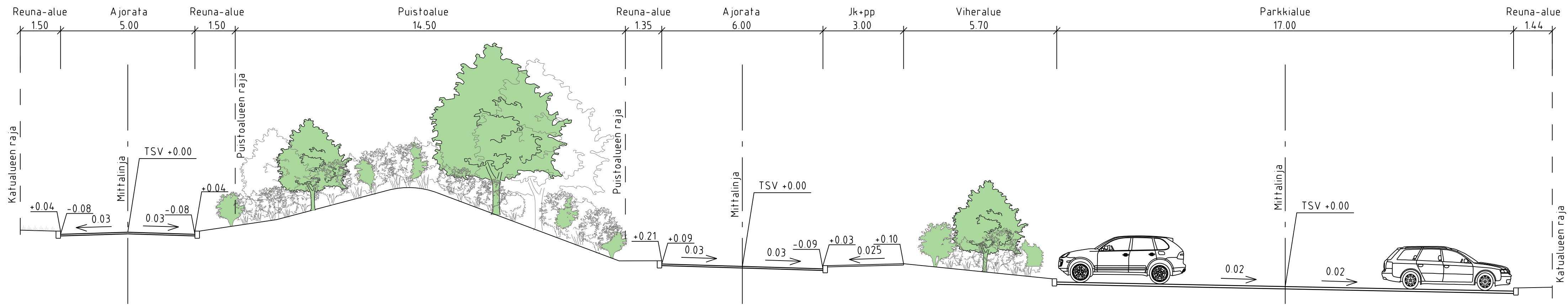
TYYPPIPOIKKILEIKKAUS A-A 1:200
