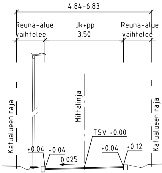
TYYPPIPOIKKILEIKKAUS A-A 1:100
